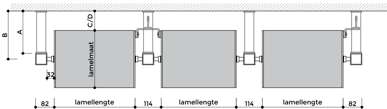
Overzicht maatvoering centraal beweegbaar (maten in mm)
