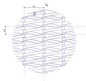
Detail H-1 (schaal 1:2)
