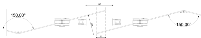
Detail H-3 (schaal 1:5)
