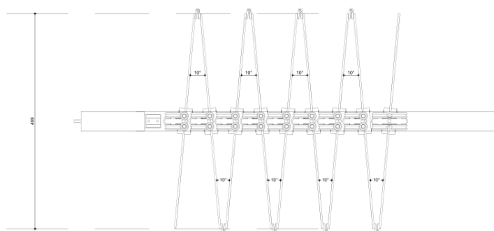
Detail H-3 (schaal 1:5)
